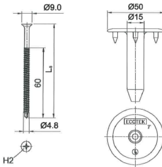
Fig. 6 – Vis EJOT DABO® TKR-4,8 + tube EJOT ECOTEK® T 50
