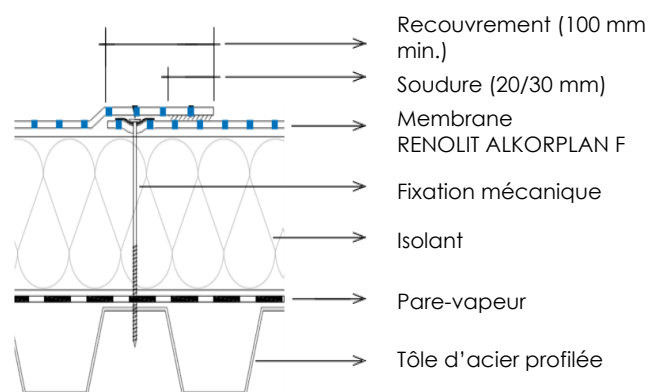
Fig. 8 – Recouvrement des lés
