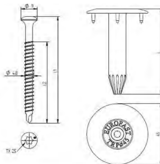
Fig. 5 – Vis VRF EUROFAST® EDS B + tube VRF EUROFAST® BTRP45
