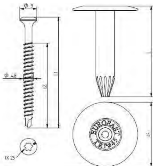
Fig. 4 – Vis VRF EUROFAST® EDS B + tube VRF EUROFAST® TRP45
